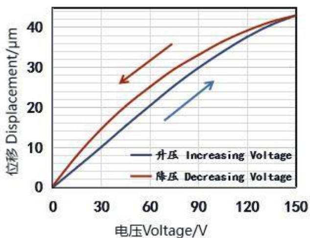
位移 Displacement(9N/20°C)
