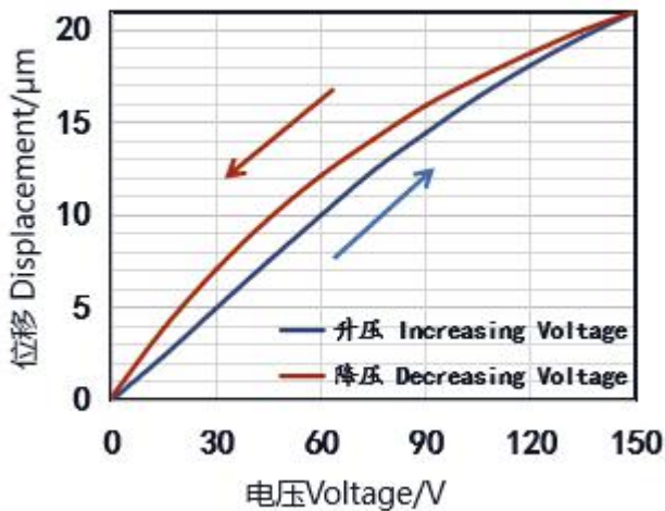
位移 Displacement(9N/20°C)
