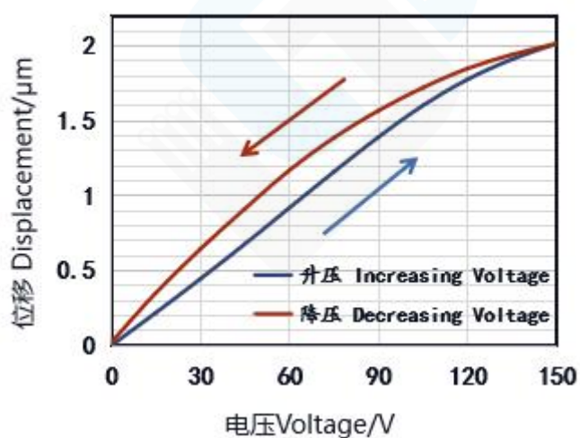
位移 Displacement(9N/20°C)
